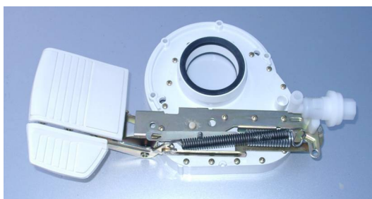
Mechanismus für Toilette AquaMagic, Starlite und Galaxy Art. Nr. 35.304.02
