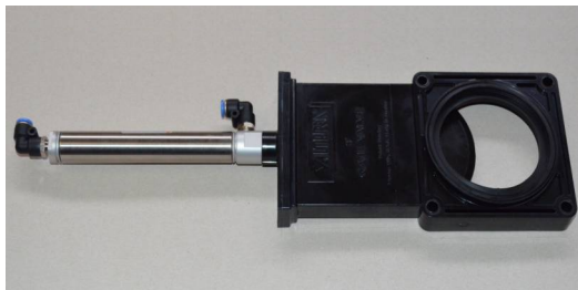
NEU z.B. für Travego Schieber druckluftbetätigt Falterra Art. Nr. 35.300.30
